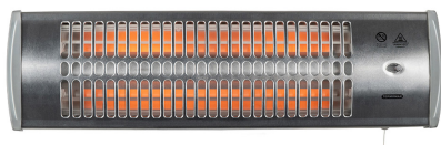
obj.č.: 1003136 TERMOMAX nástěnný křemenný ohřívač 2stupňová regulace výkonu: 600/1200 W 2 křemenná topná tělesa bezdotykové zapínání šňůrkou odolnost proti vodě a prachu IP24
